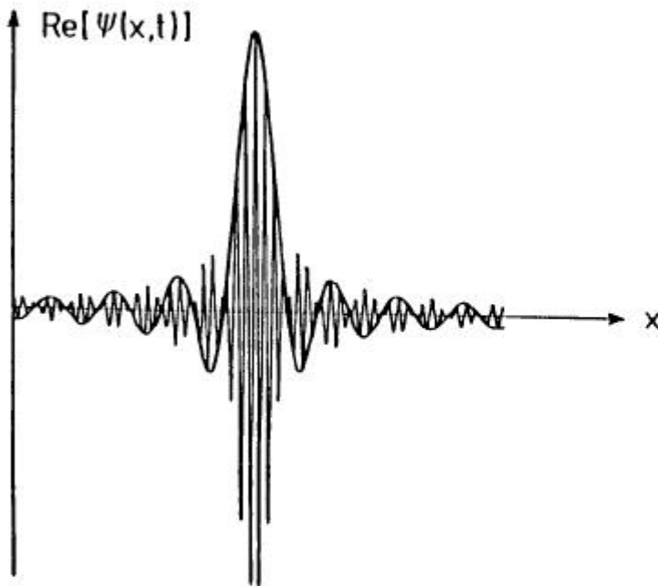
Abb. 7.3. Der Realteil von \psi(x, t) als Funktion des Orts x . Die rasche Oszillation wird durch \cos(k_0 x - \omega_0 t) , t fest, beschrieben, die Einhüllende durch
