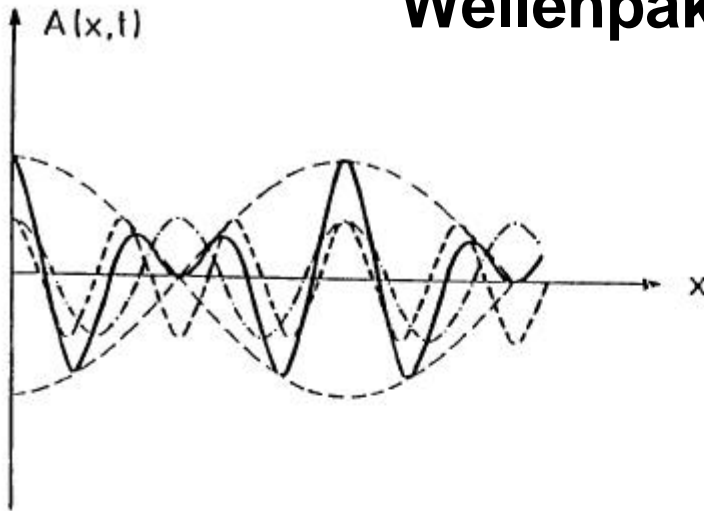
Abb. 7.2. Überlagerung zweier Wellen gleicher Amplitude. Grundwelle 1: strichpunktiiert. Grundwelle 2: gestrichelt, gleiche Amplitude wie Grundwelle 1. Gesamtwelle A : ausgezogen. Einhüllende \cos(\Delta kx - \Delta \omega t) , t fest, wieder gestrichelt
