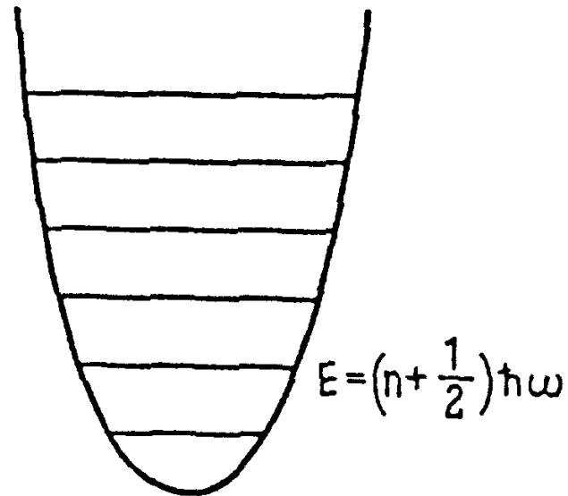
harm. Oszillator
