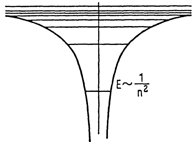
Coulomb
